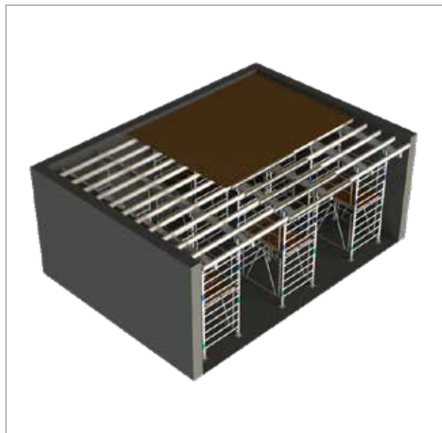
- Étalement pour dalle coulée en place avec AL200 sur tours A120.
